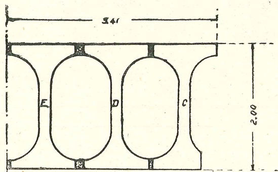
b) SEMI-SECCION VIGAS TRAMO CORTO
