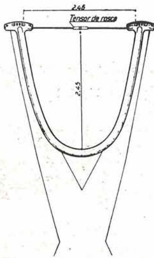
SECCIÓN TRANSVERSAL
