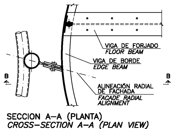
Figura 18. Croquis de unión de estructura interior con tubos de fachada
