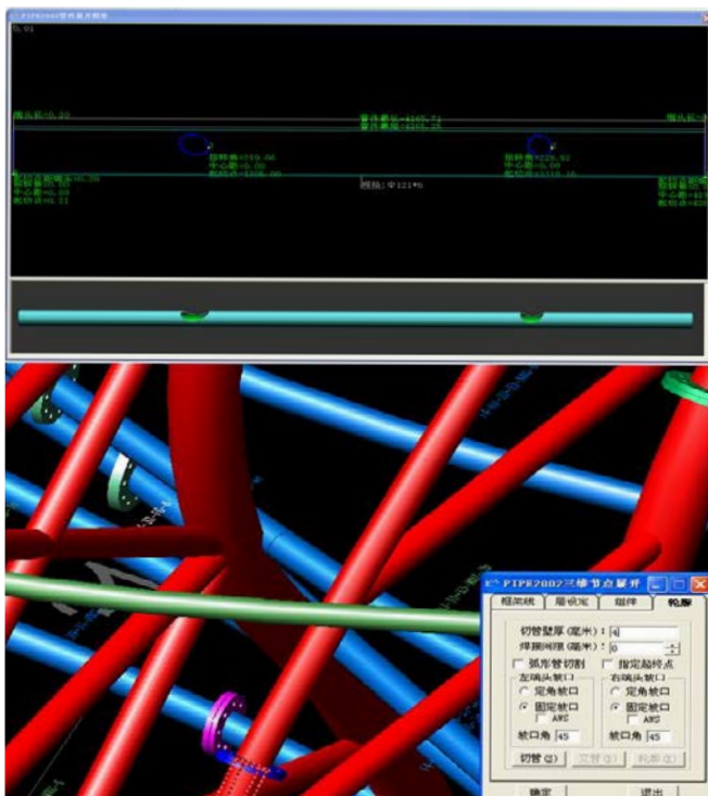
Figura 16. Interfaz del software desarrollado para el corte en intersección excéntrica de barras curvas Figure 16. Interface of the software developed for automatic cut of curved tubes
