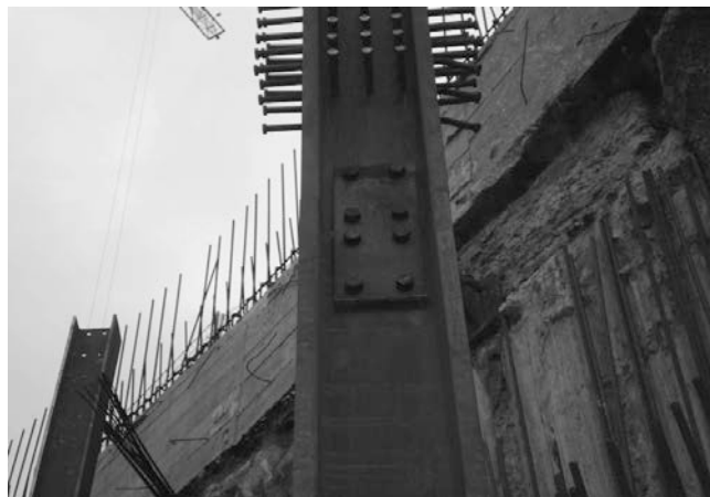
Figura 21. Pilares mixtos. Conexión entre tramos consecutivos
