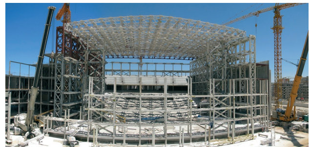
Figura 14. Vista de la estructura del auditorio durante su construcción
