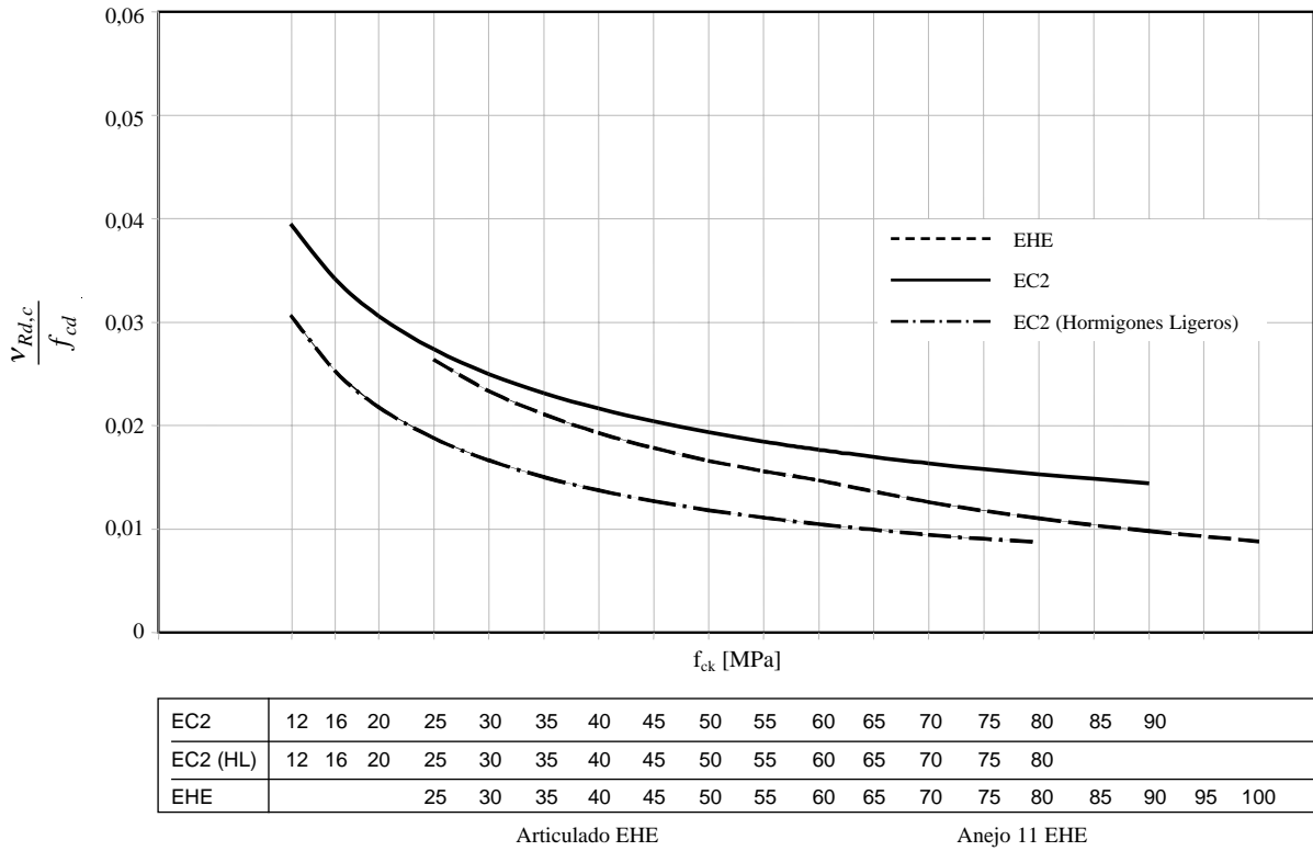
Figura 15.a) Evolución de la resistencia a punzonamiento del hormigón en elementos con armadura transversal con la resistencia característica a compresión en probeta cilíndrica. d=0.25 m, ρl=0.5%.
