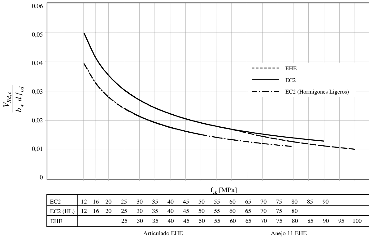
Figura 12.e). Evolución de la resistencia a cortante de elementos sin armadura transversal con la resistencia característica a compresión en probeta cilíndrica. h=1.0 y ρ l =1.0%.
