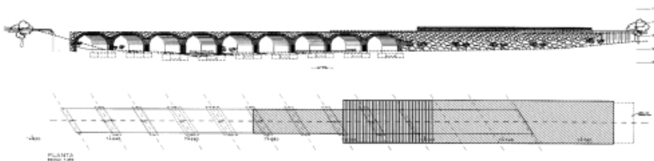
Figura 8. Proceso constructivo planteado para la ampliación transversal de la estructura de la Rambla primera en el P.K. 7+700. Llíria-Casinos.
