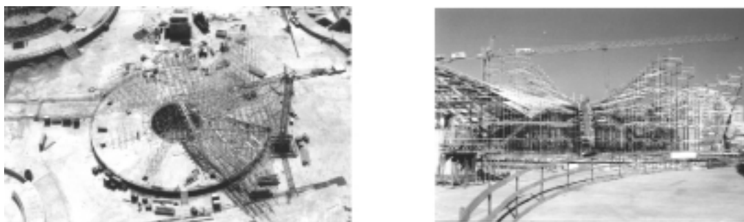
Figura 3. Cimbrado.
