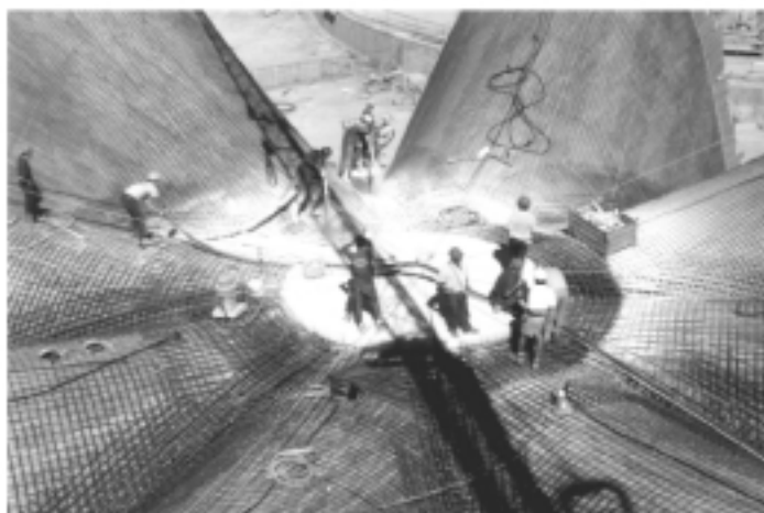
Figura 11. Hormigón proyectado de clave y nervios.
