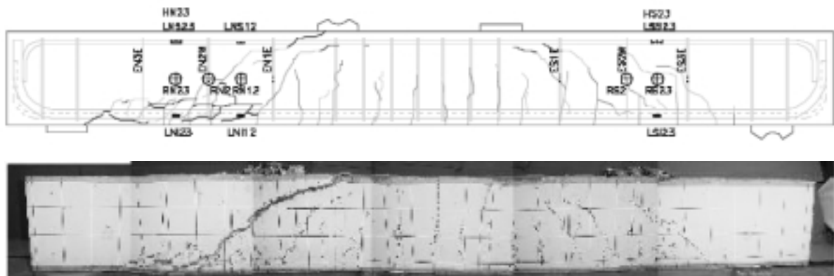
Figura10.- Diagrama de fisuras y vista real de la fisuración y rotura de la viga V24HR.
