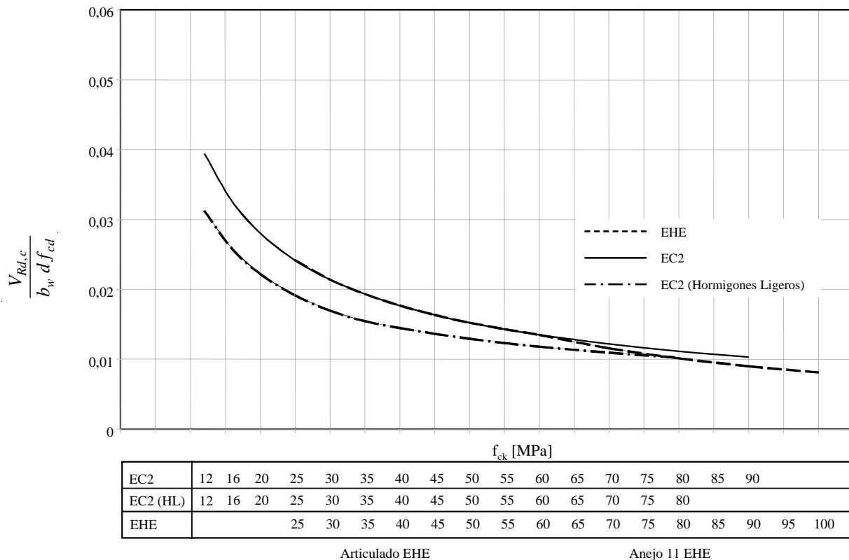
Figura 12.d). Evolución de la resistencia a cortante de elementos sin armadura transversal con la resistencia característica a compresión en probeta cilíndrica. h=1.0 y ρ t =0.5%
