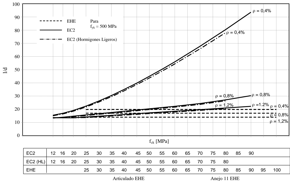
Figura 18. Límites de esbeltez para hormigones de distintas resistencias. ρ constante.
