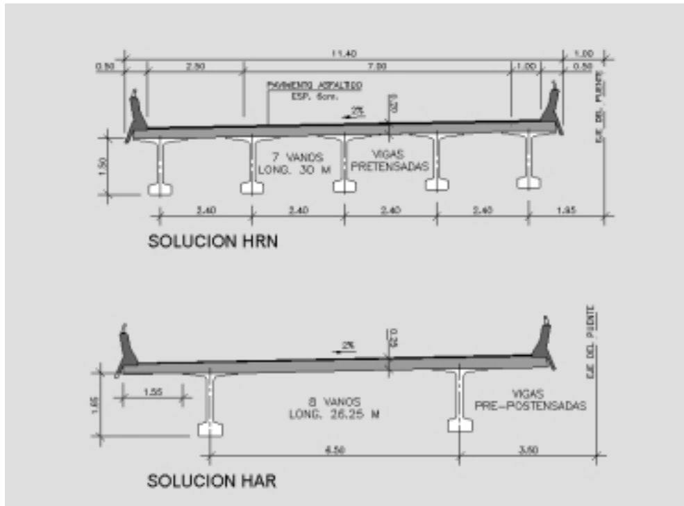
Figura 3: Comparación entre tableros con vigas de HRN y de HAR. P. del Guadalete.
