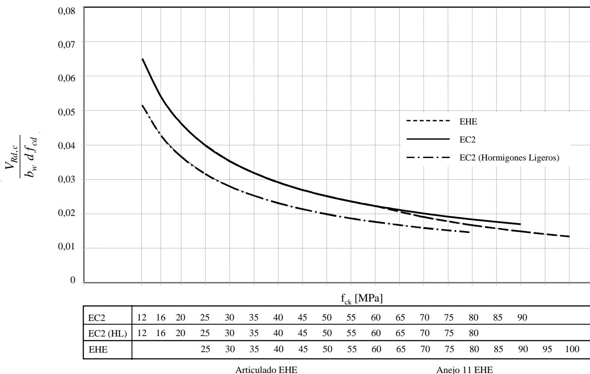
Figura 12.b). Evolución de la resistencia a cortante de elementos sin armadura transversal con la resistencia característica a compresión en probeta cilíndrica. h=0.25 y ρ l =1.0%.
