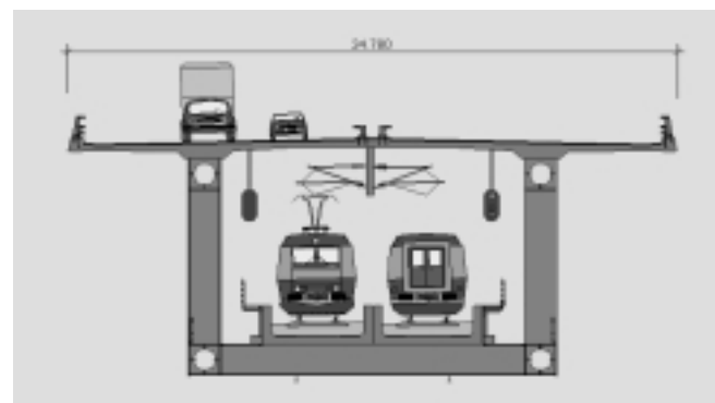
Figuras 15 y 16: Instalaciones de fabricación y sección del tablero. P. de Oresund.
