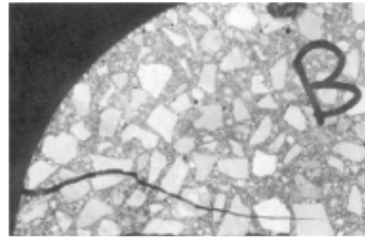
Figura 1: Fisura en HAR que cruza los áridos. Extraída de "La EHE explicada por sus autores" (1).
