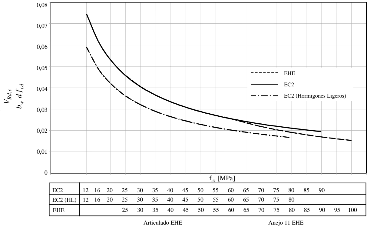
Figura 12.c). Evolución de la resistencia a cortante de elementos sin armadura transversal con la resistencia característica a compresión en probeta cilíndrica. h=0.25 y ρ t =1.5%.
