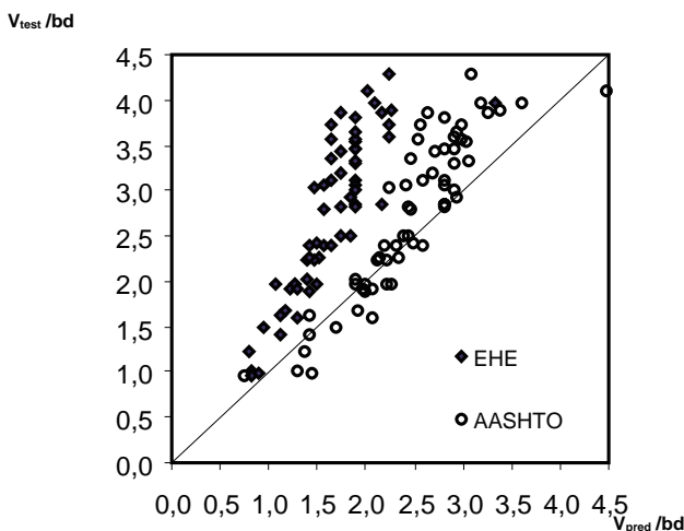
Figura 19: Comparación resultados experimentales con los obtenidos al aplicar la Instrucción EHE y el código AASHTO, basado en la teoría modificada del campo de compresiones.
