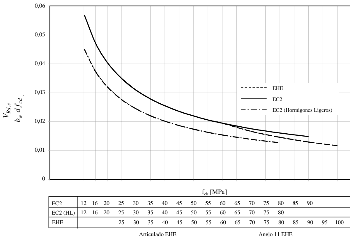
Figura 12.f). Evolución de la resistencia a cortante de elementos sin armadura transversal con la resistencia característica a compresión en probeta cilíndrica. h=1.0 y ρ l =1.5%.
