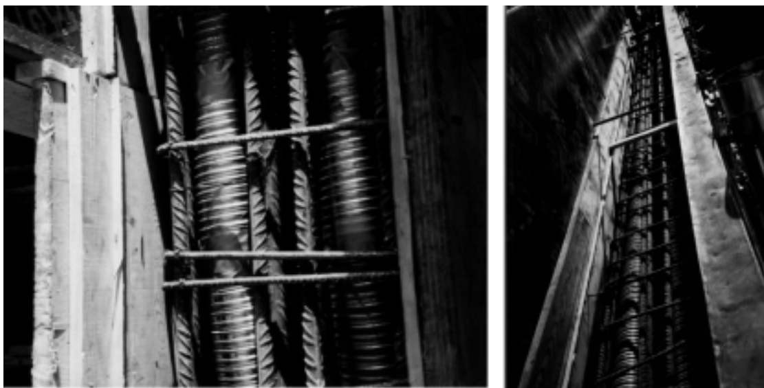
Foto 3. Vista desde la parte superior del encofrado, donde se observa la alta densidad de refuerzo en los muros postensados.
