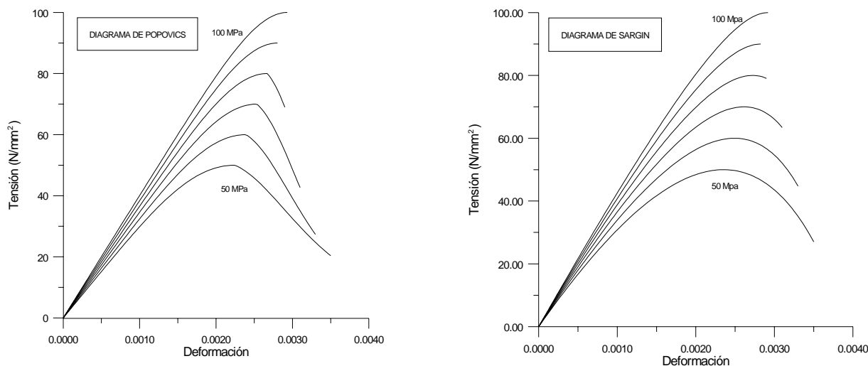
Figura 2.: Diferencia de rigidez entre áridos y pasta de cemento en HC y HAR (fip-CEB Working Group on HSC, 1990).
