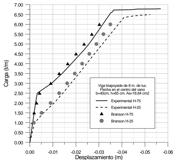
Figura 20: Influencia del tipo de hormigón en la deformabilidad de una viga.
