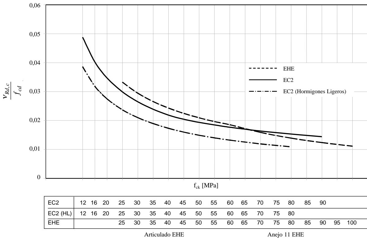
Figura 15.b) Evolución de la resistencia a punzonamiento del hormigón en elementos con armadura transversal con la resistencia característica a compresión en probeta cilíndrica. d=0.25 m, ρl=1.0%.
