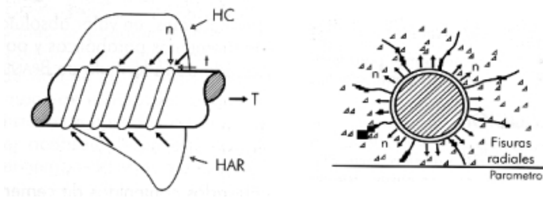
Figura 8: Distribución de tensiones de adherencia y fisuración radial en anclajes de armaduras pasivas en HAR (Extraída de "La Instrucción EHE explicada por sus autores")
