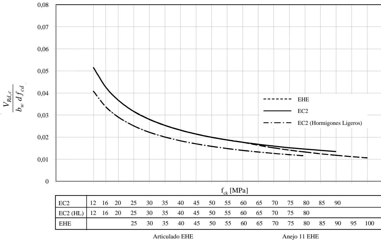
Figura 12.a). Evolución de la resistencia a cortante de elementos sin armadura transversal con la resistencia característica a compresión en probeta cilíndrica. h=0.25 y ρ l =0.5%.
