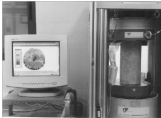
Fotografía n.º 2. Ensayo de una probeta con medida de la distribución de presiones en el refrentado.
