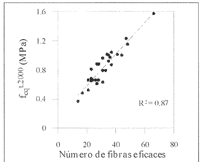
Figura 12. Variación de los valores de f_{eq}^{1,2000} con el número de fibras eficaces.
