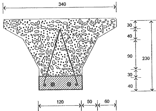
b) Viguetas armada
