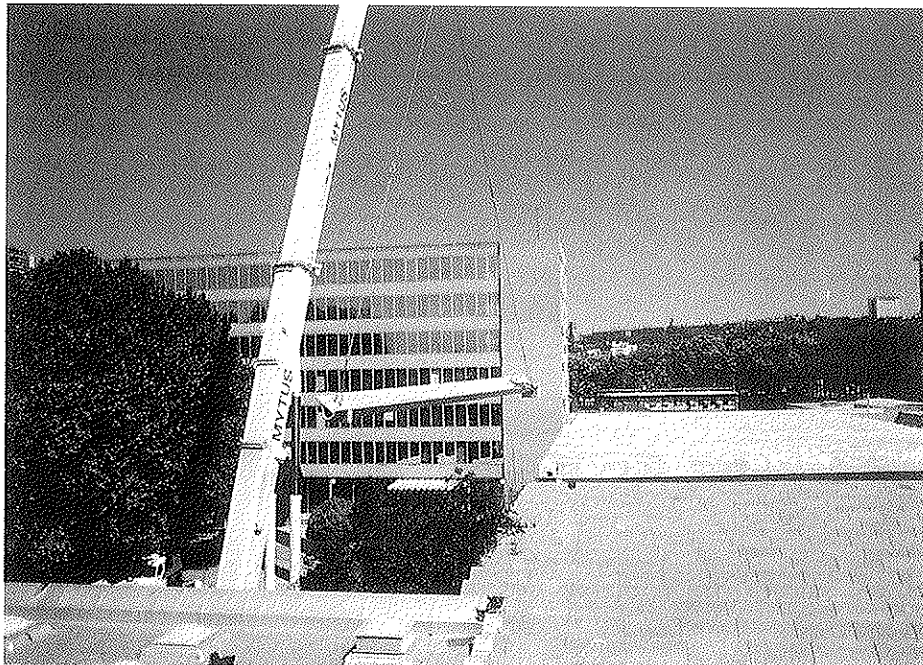
Foto 17. Vista superior de la cubierta durante la sustitución. Puede apreciarse la ligera pendiente transversal (longitudinal a las vigas) que se dió en la nueva cubierta.
