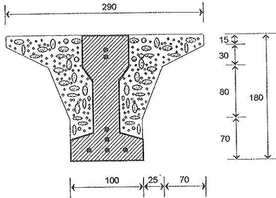
a) Viguetas pretensada
