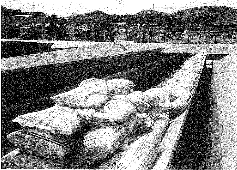
Foto 12. Aspecto parcial de la prueba de carga de una viga, durante su acopio en fábrica. El control de deformaciones se llevó a cabo mediante flexímetros fijados al suelo.
