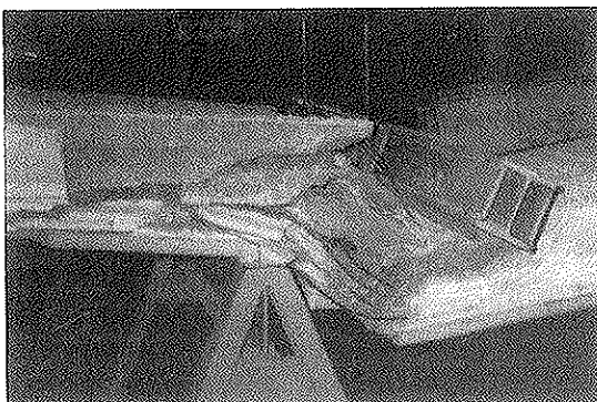
Forjado pretensado con refuerzo inferior. Rotura por cortante en la sección de aplicación de la carga.
