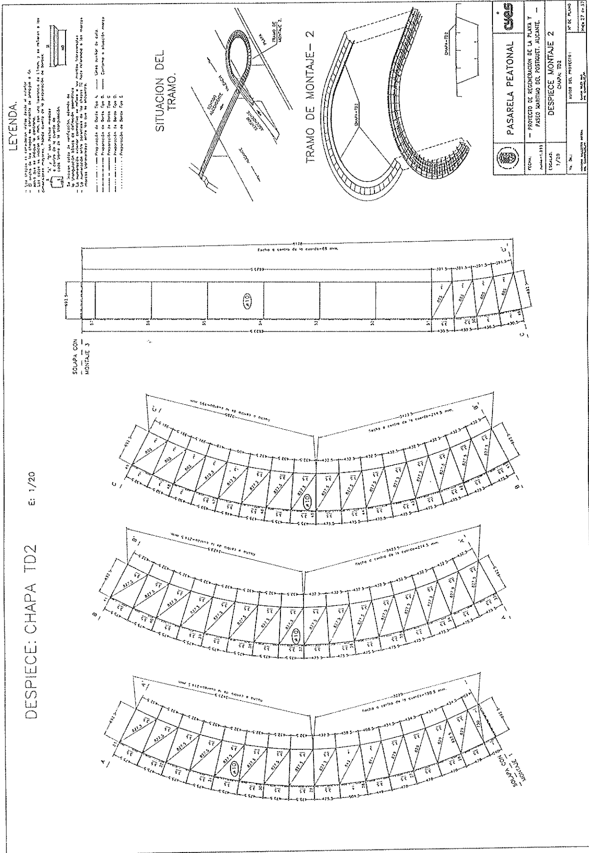
Fig. 9. Plano tipico de despiece de chapas.
