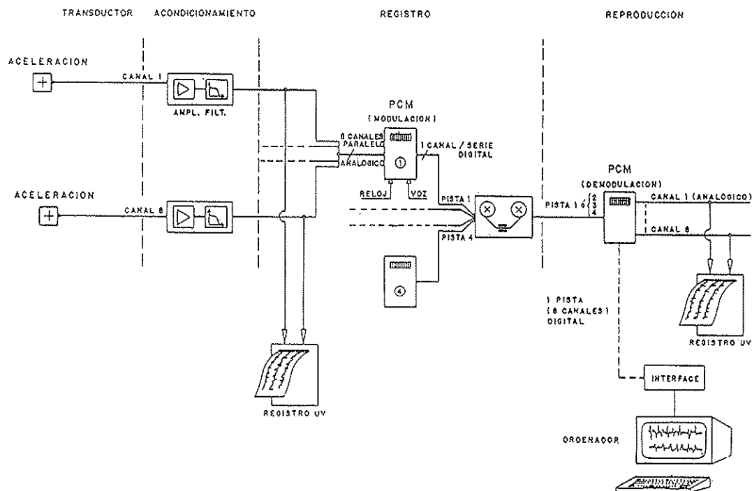
Fig. 6. Sistema de registro y reproducción de las señales.
