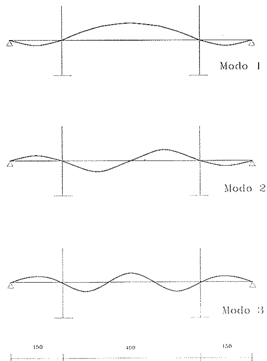
Fig. 9. Ranre: Tres primeros modos de flexión vertical.
