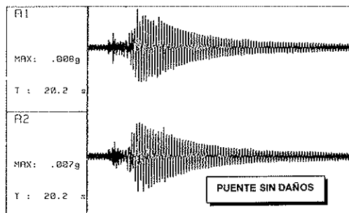
Fig. 10. Auscultación dinámica.
