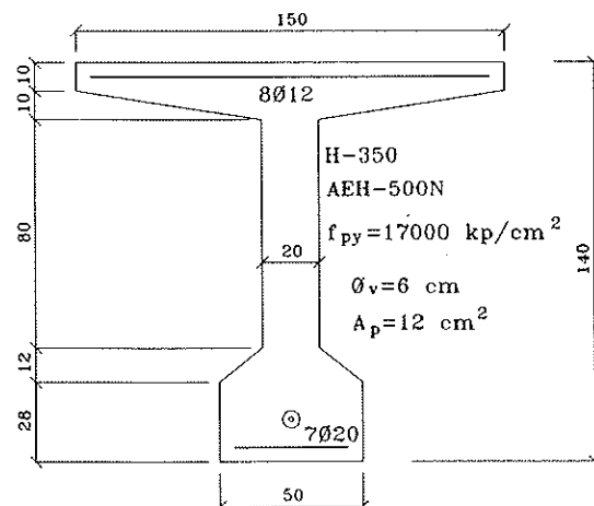
Figura 8. Sección transversal.
