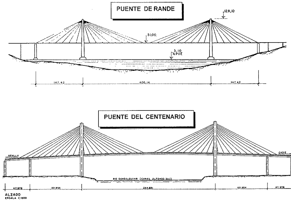
Fig. 1. Alzados.
