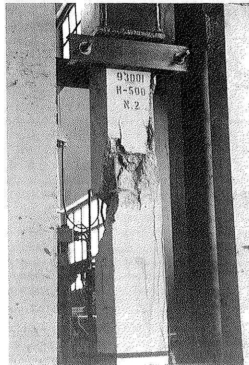
Foto 8. Rotura de un pilar de hormigón H-500.
