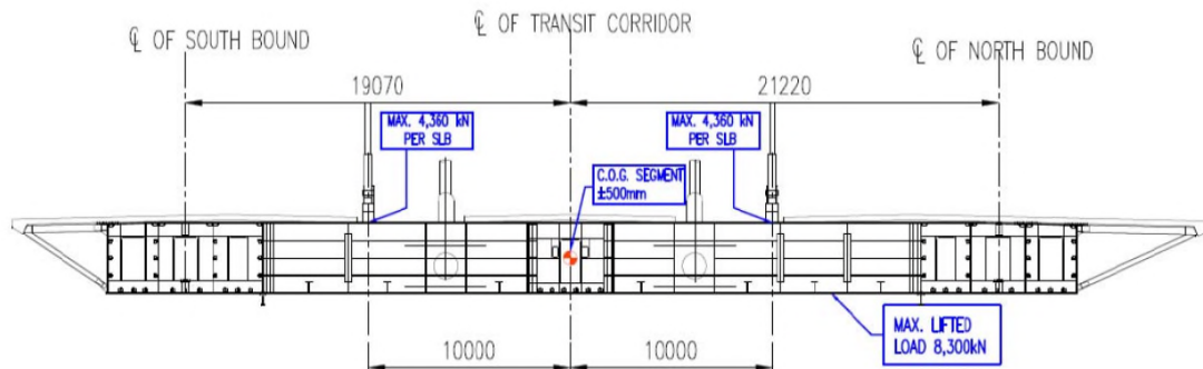
Figura 33. Disposición de puntos de cogida en la dovela. Puente de Champlain.
