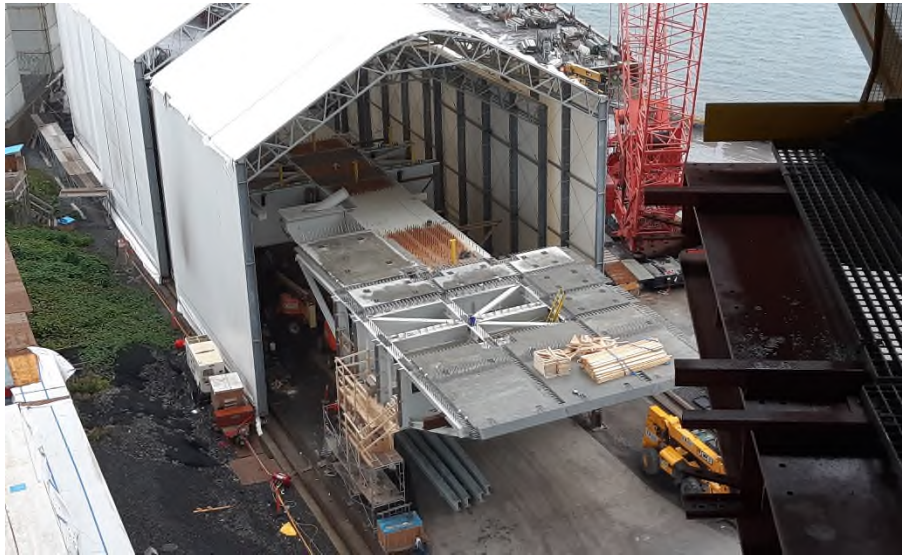
Figura 29. Vista de ½ dovela tipo. Puente de Champlain.
