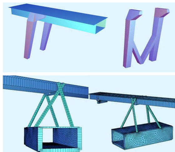
Figura 4. Alternativas estudiadas durante la fase de diseño.
