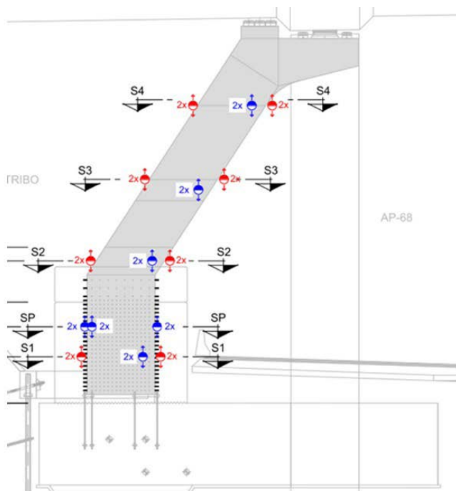
Figura 13. Secciones de control y ejemplo de galga instalada.
